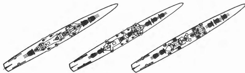
WICHITA
